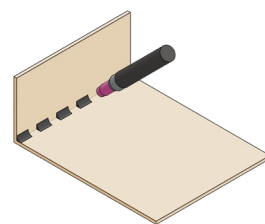
▲斷續焊
